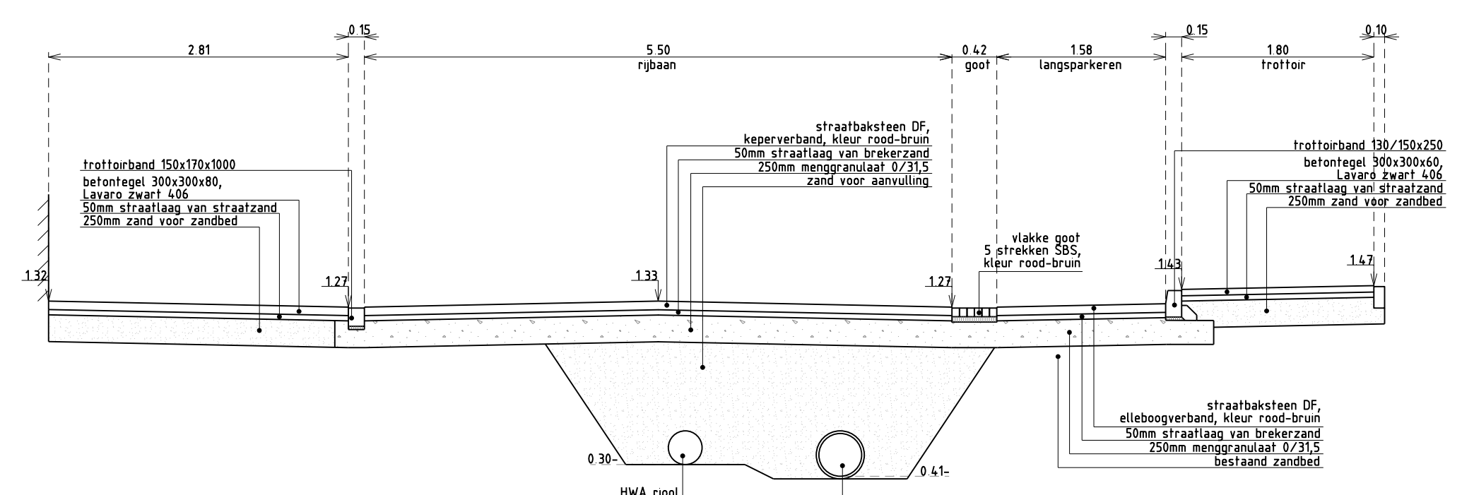
DWARPROFIEL A-A
